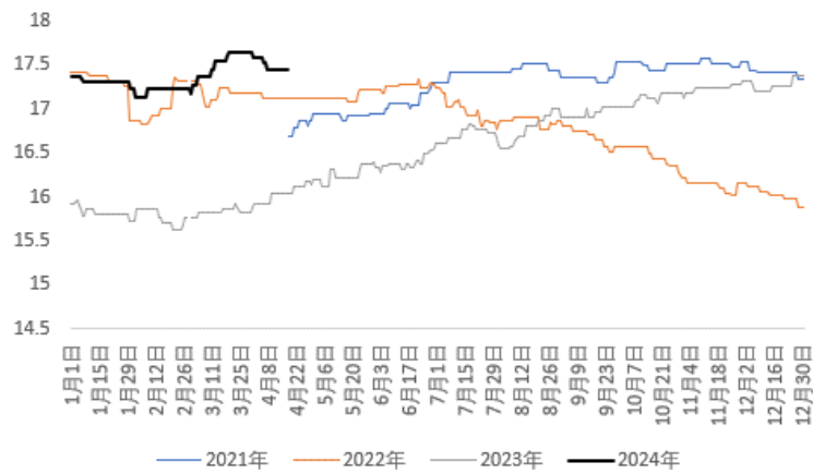
图表 5: 浮法玻璃日熔量 (万吨)
